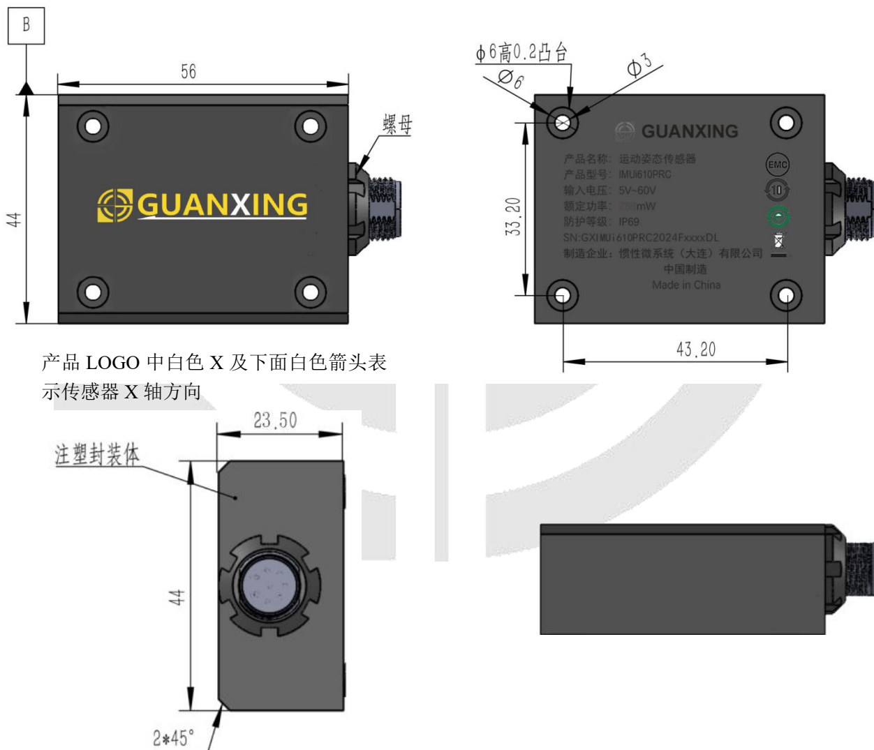
图 7 传感器主体各部位尺寸
