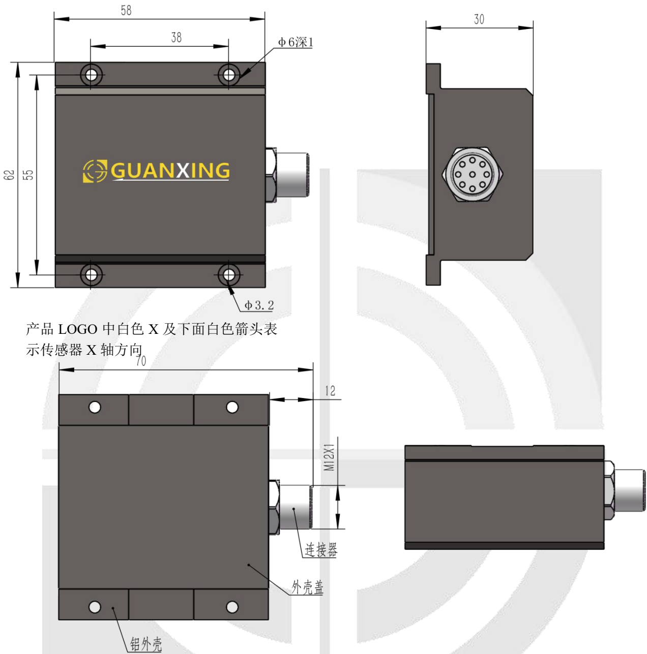
图 6 传感器主体各部位尺寸
