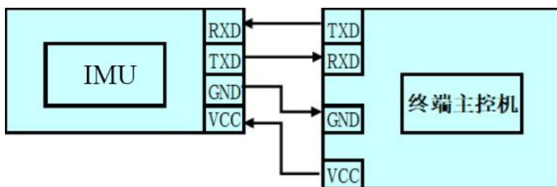
图5 串口传输示意图
