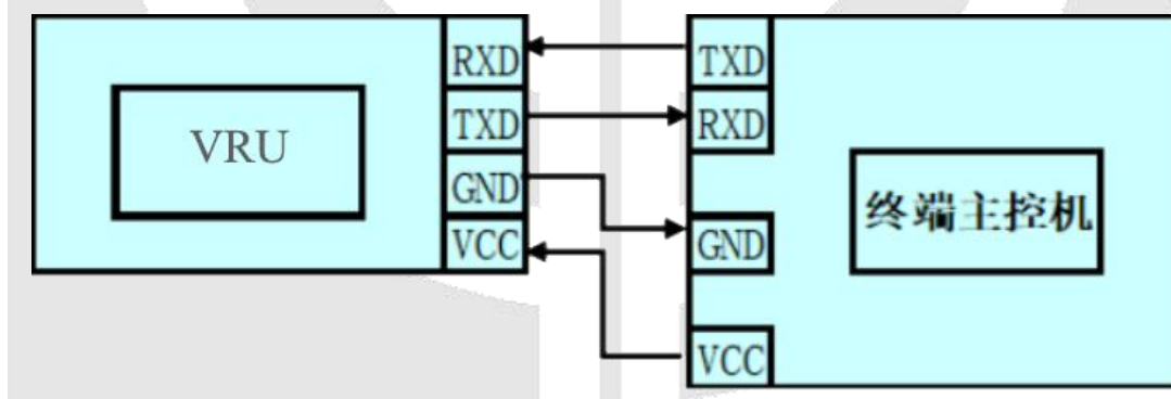
图5 串口传输示意图
