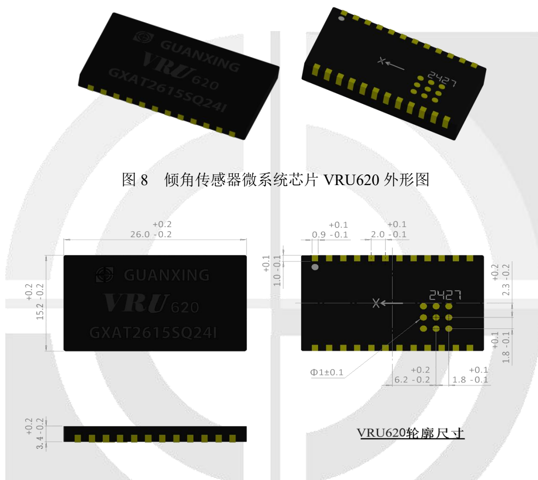
图9 倾角传感器微系统芯片 VRU620封装尺寸
