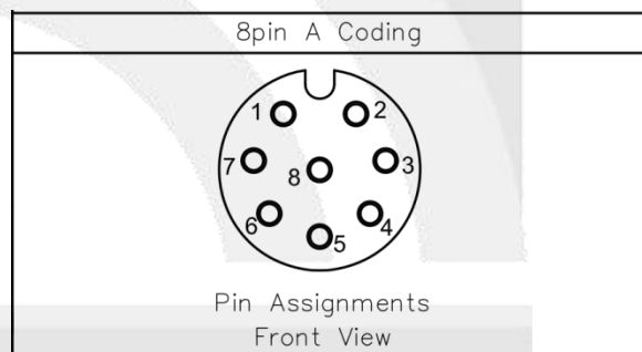
图 8 航空连接器引脚定
