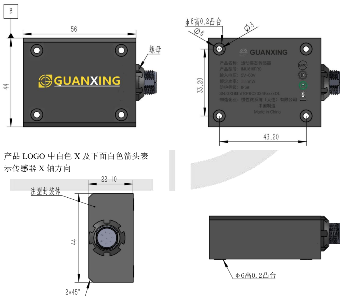
图 6 传感器主体各部位尺寸
